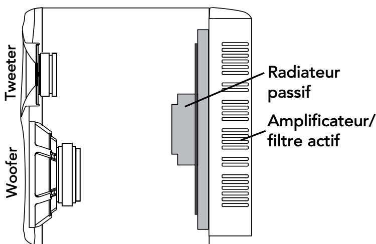
Figure 1. - Vue en coupe du moniteur HR624 MK2
