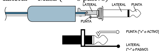
Conector TS de 6,3 mm
