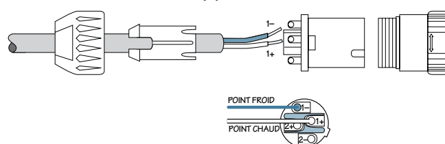
Connecteur Speakon
